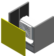
Séparation de l'air
